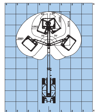
Option 3D: Drehung des Schwenkarms
